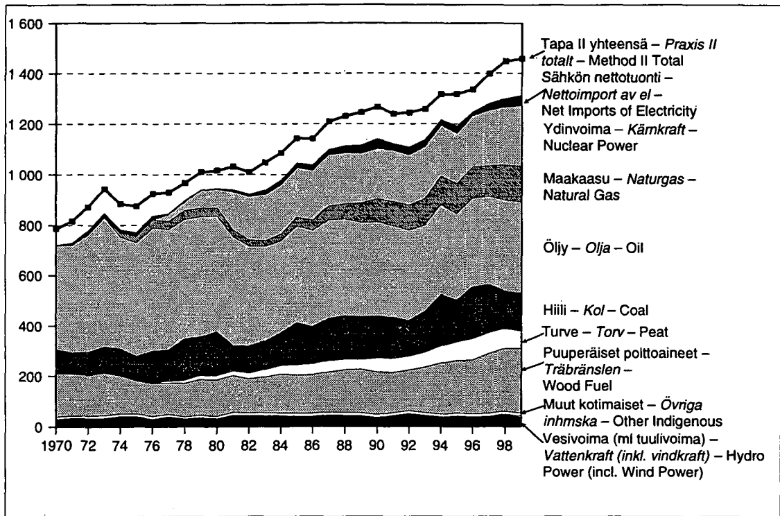
Kuva – Figur – Figure 1 Energian kokonaiskulutus energialähteittäin 1970–1999, PJ Totalförbrukning av energi enligt energikälla 1970–1999, PJ Total Energy Consumption by Energy Source 1970–1999, PJ
