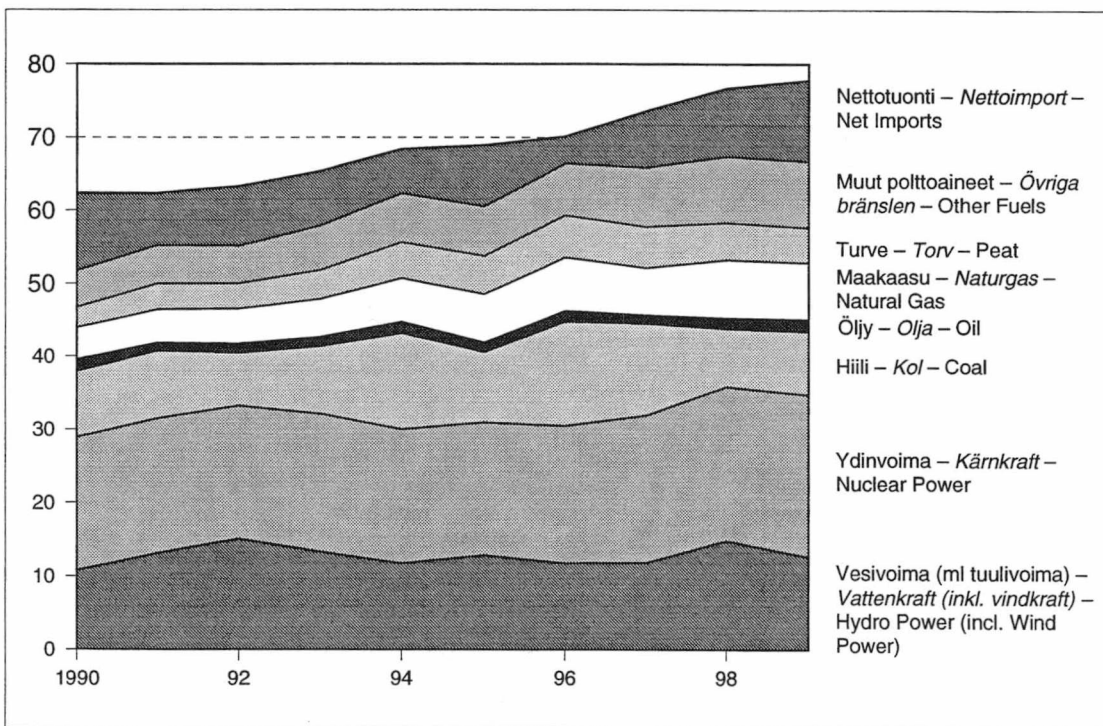
Kuva – Figur – Figure 4 Sähköntuotanto energialähteittäin 1990–1999, TWh Produktion av el enligt energikälla 1990–1999, TWh Electricity Generation by Energy Source 1990–1999, TWh
