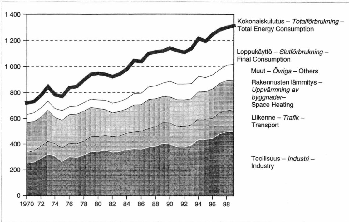
Kuva – Figur – Figure 3 Energian käyttö loppukulutussektoreittäin 1970–1999, PJ Förbrukning av energi enligt slutförbrukningssektor 1970–1999, PJ Final Energy Consumption by End-Use Sector 1970–1999, PJ
