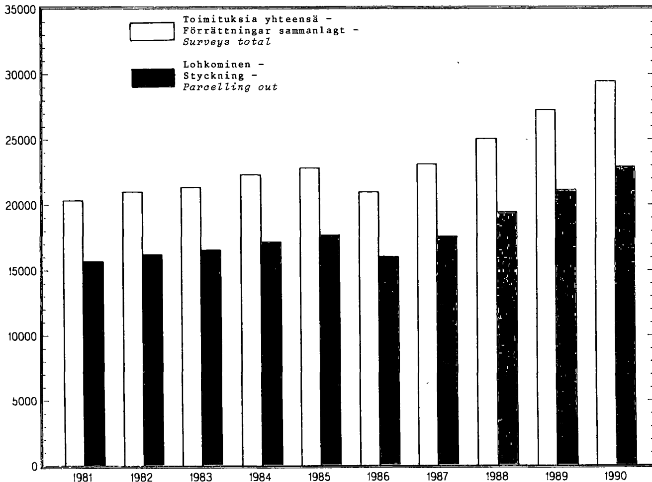
KUVIOT 5-7. VUOSINA 1981-1990 LOPPUUNSAATETUT MAANMITTAUSTOIMITUKSET FIGURER 5-7. UNDER ÅREN 1981-1990 SLUTFÖRDA LANTMÄTERIFÖRRÄTTNINGAR FIGURES 5-7. SURVEYS COMPLETED IN 1981-1990
