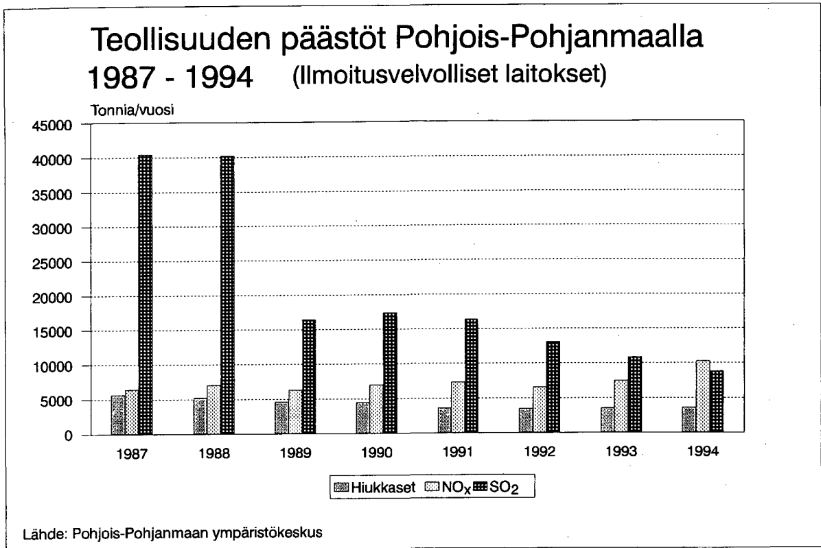
Kuva 123. Teollisuuden päästöt Pohjois-Pohjanmaalla 1987 - 1994.
