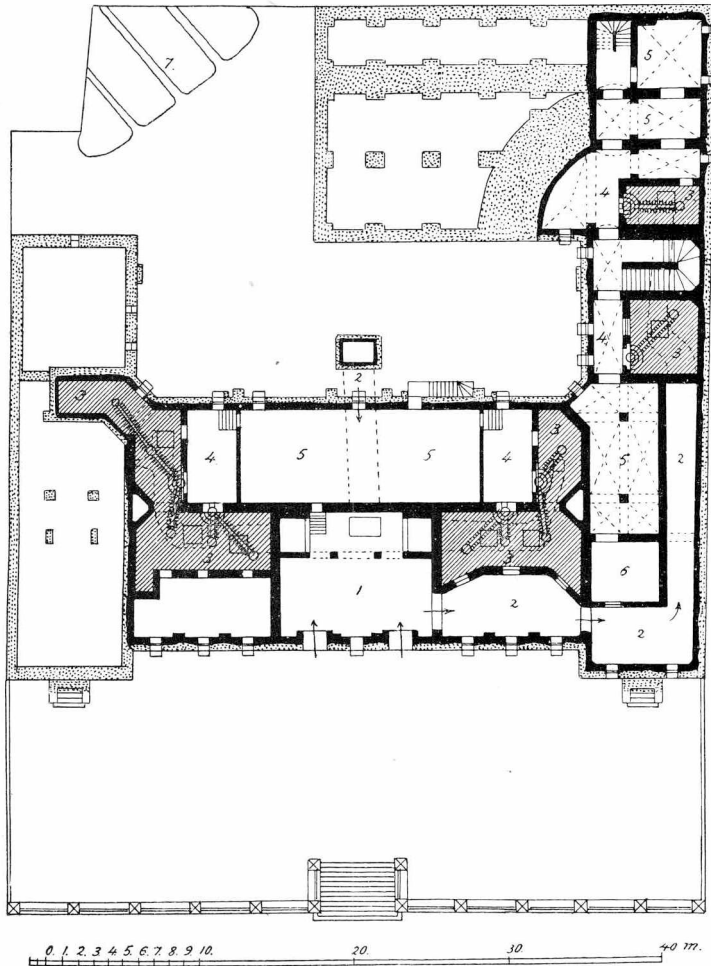
KÄLLARVÅNINGEN.
