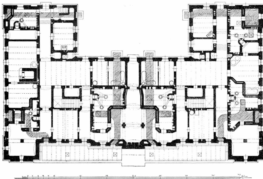
PLAN AF KÄLLAR- VÅNINGEN.
