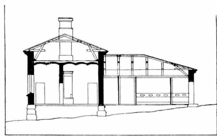
LEIKKAUS.
