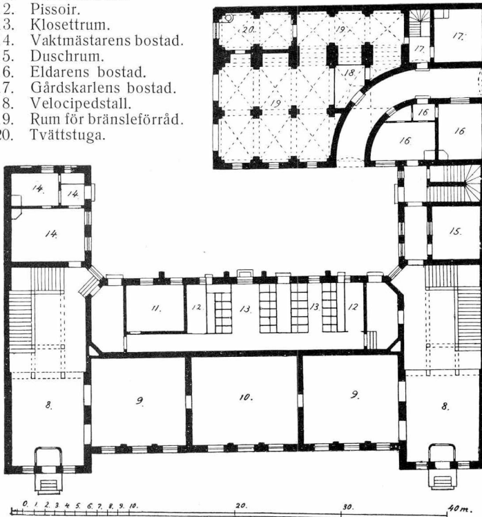
1 VÅN. 1 NEN KERROS.
