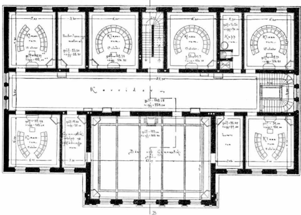
PLAN AF 1 a VÅNINGEN. 1 n KERR. POHJA.
