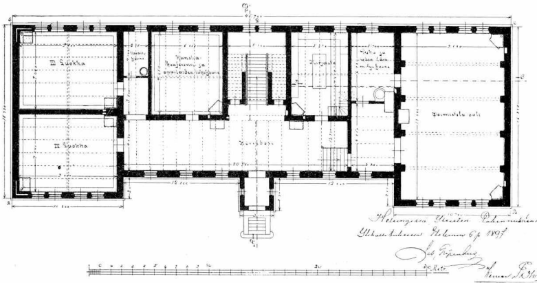
POHJAKERROS. — BOTTENPLAN.
