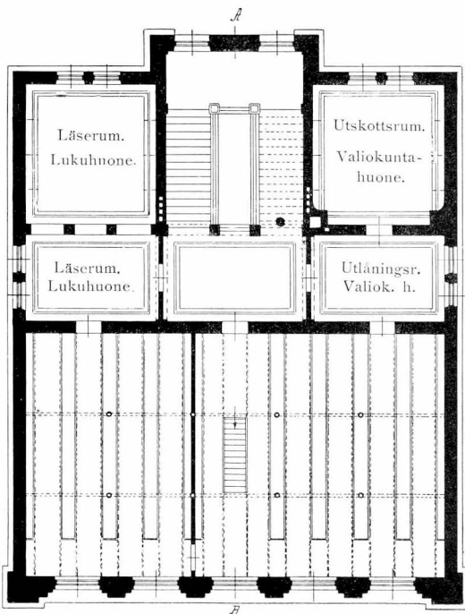
PLAN AF 1 STA VÅNINGEN. ENSIMÄISEN KERROKSEN POHJAPIIRROS.
