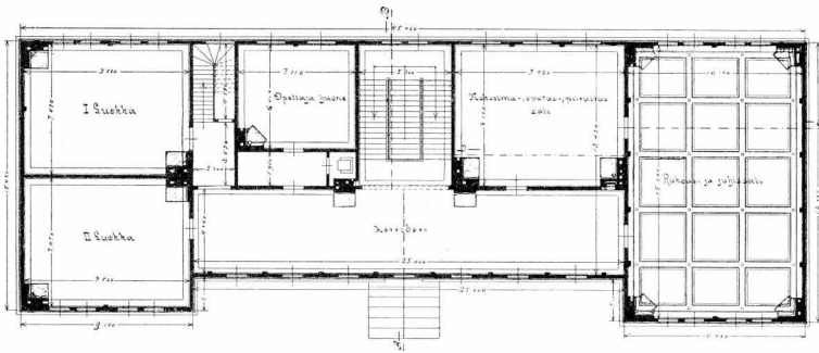
2 SEN KERR. POHJA. — PLAN AF 2 Å VÅNINGEN.
