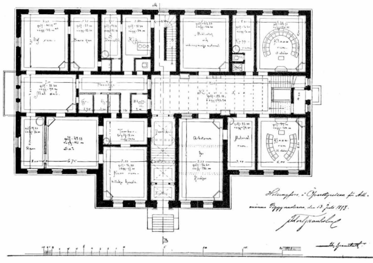
PLAN AF 1 a VÅNINGEN. 1 n KERR. POHJA.
