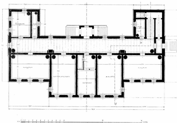
BOTTENPLAN. — POHJAKERROS.
