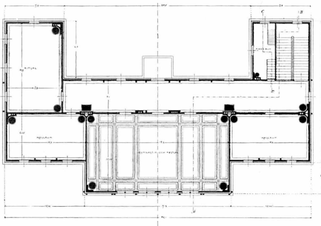
PLAN AF 2 RA VÅNINGEN. — 2 SEN KERR. POHJA.
