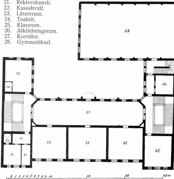
2 VÅN. 2 NEN KERROS.
