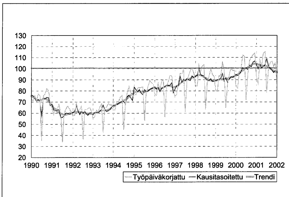
Kuvio 9. Muu metalliteollisuus TOL met -DL, teollisuustuotannon volyymi-indeksi 1990 - 2002, 2000=100
