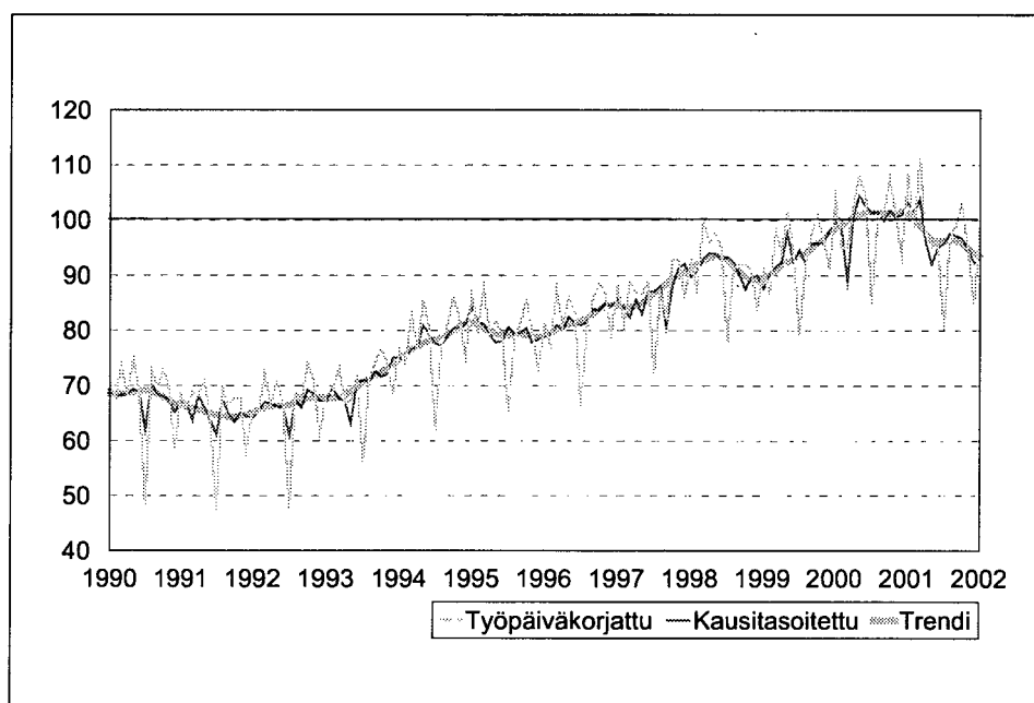
Kuvio 8. Kemian teollisuus TOL 23-25, teollisuustuotannon volyymi-indeksi 1990 - 2002, 2000=100
