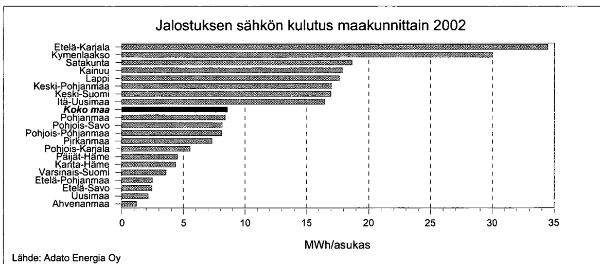
Kuva 184. Jalostuksen sähkön kulutus maakunnittain 2002.
