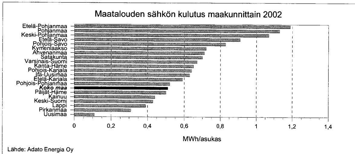
Kuva 186. Maatalouden sähkön kulutus maakunnittain 2002.
