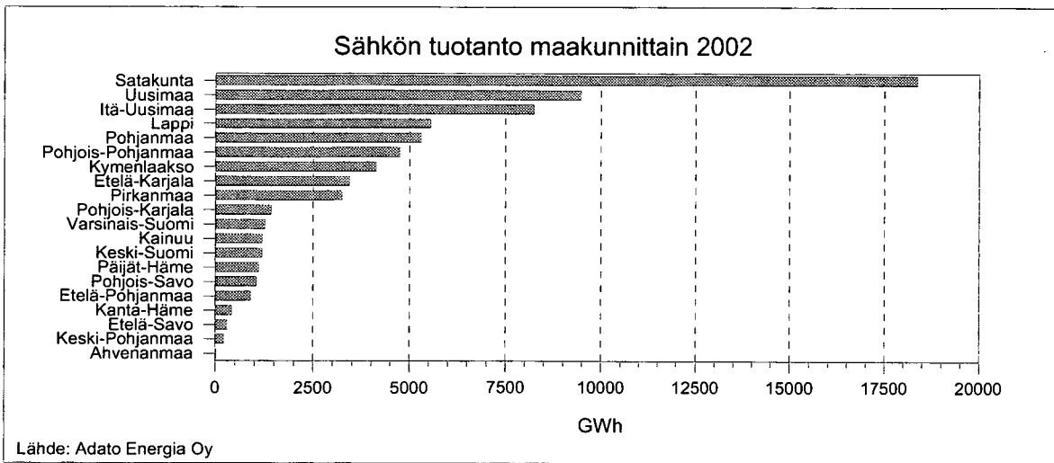
Kuva 180. Sähkön tuotanto maakunnittain 2002.
