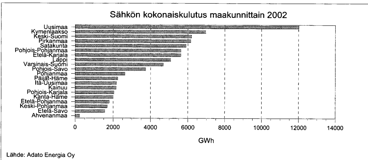
Kuva 182. Sähkön kokonaiskulutus maakunnittain 2002.
