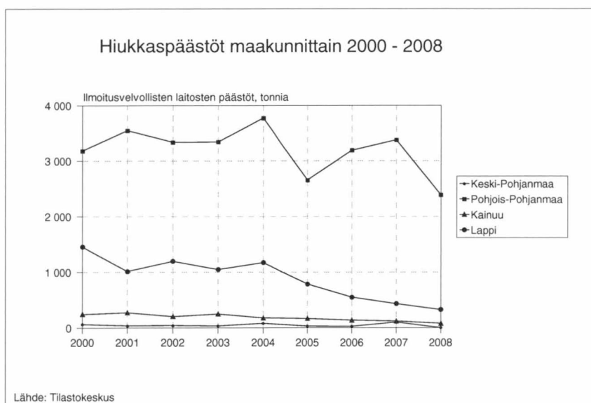
Kuva 15.5. Hiukkaspäästöt maakunnittain 2000–2008.
