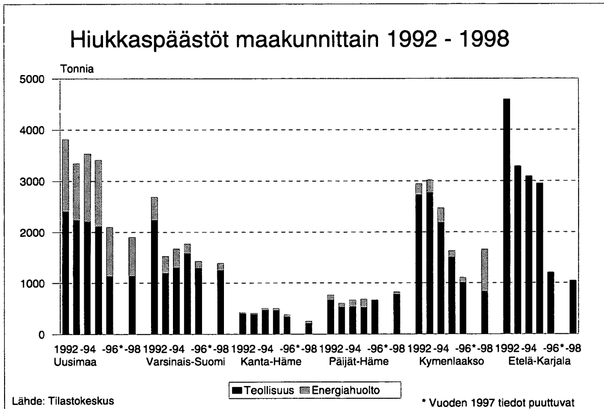
Kuva 111. Hiukkaspäästöt maakunnittain 1992 - 1998.
