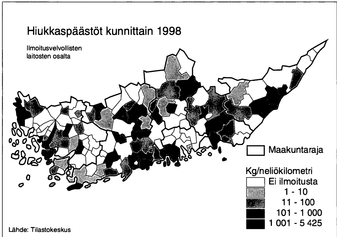
Kuva 114. Hiukkaspäästöt kunnittain 1998.
