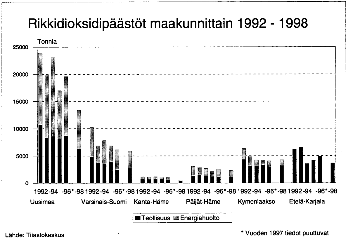
Kuva 110. Rikkidioksidipäästöt maakunnittain 1992 - 1998.
