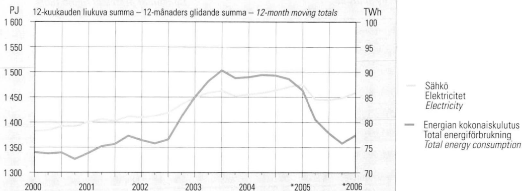
Energian kokonaiskulutus (PJ) ja sähkönkulutus (TWh) Total energiförbrukning (PJ) och elförbrukning (TWh) Total energy consumption (PJ) and electricity consumption (TWh)
