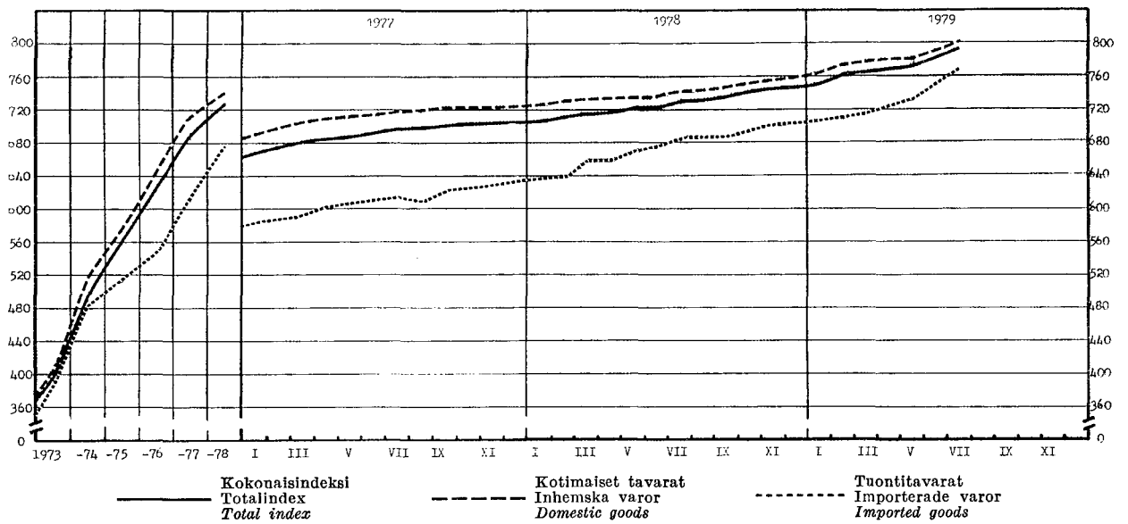
Rakennuskustannusindeksi — Byggnadskostnadsindex — Building cost index (1973 = 100) (Lähde: Taulu 31 — Källa: Tabell 31)
