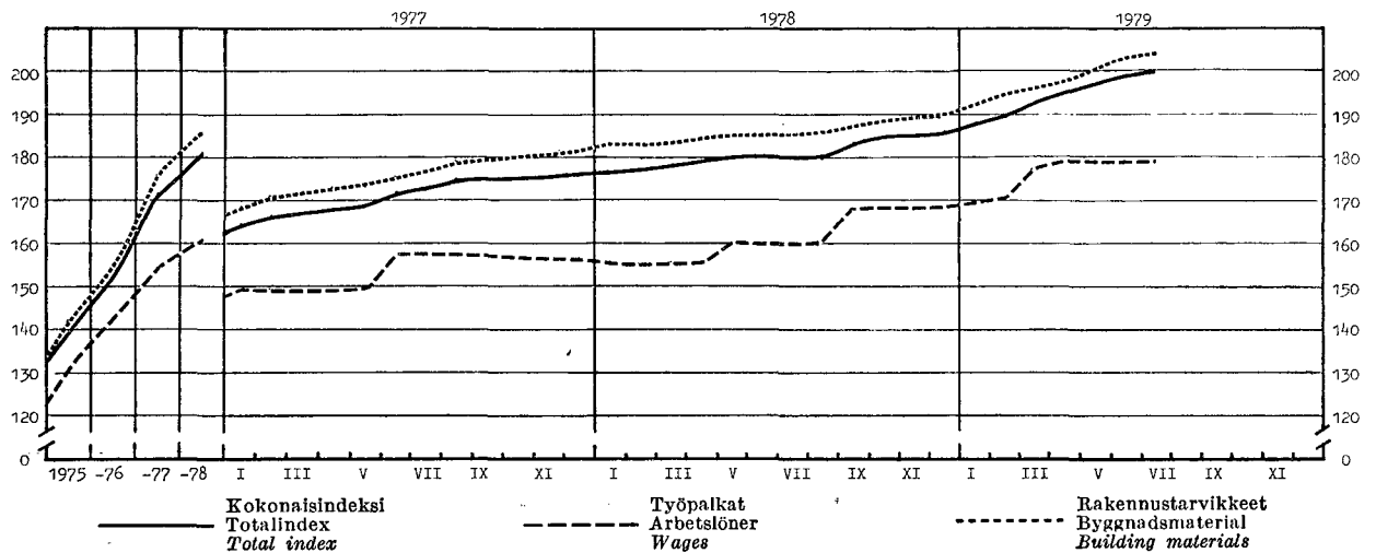
Rakennuskustannusindeksi — Byggnadskostnadsindex — Building cost index (1973 = 100) (Lähde: Taulu 31 — Källa: Tabell 31)
