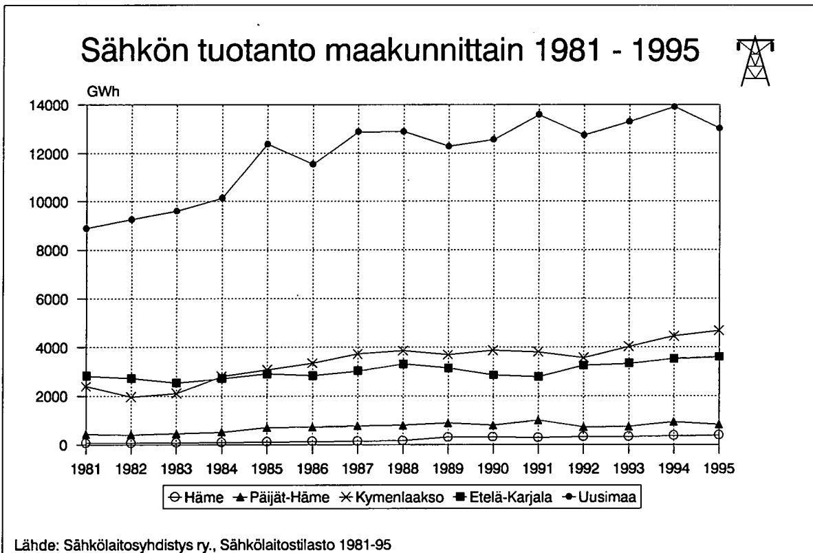
Kuva 117. Sähkön tuotanto maakunnittain 1981 - 1995.
