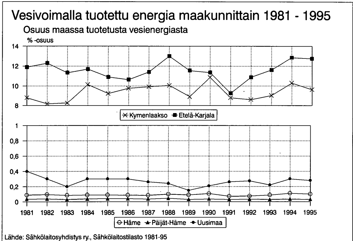
Kuva 118. Vesivoimalla tuotettu energia maakunnittain 1981 - 1995.
