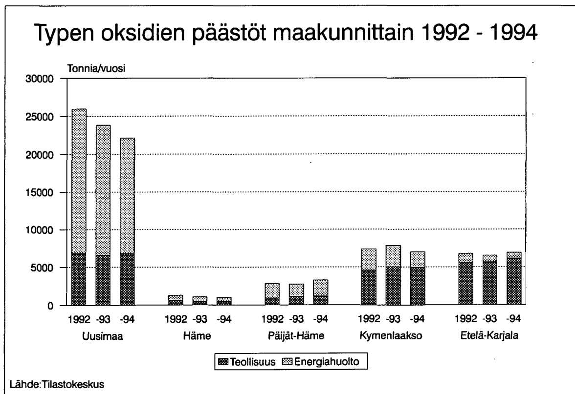
Kuva 123. Typen oksidien päästöt maakunnittain 1992 - 1994.
