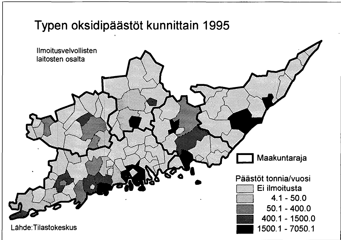
Kuva 126. Typen oksidipäästöt ( \text{NO}_x ) kunnittain 1995.
