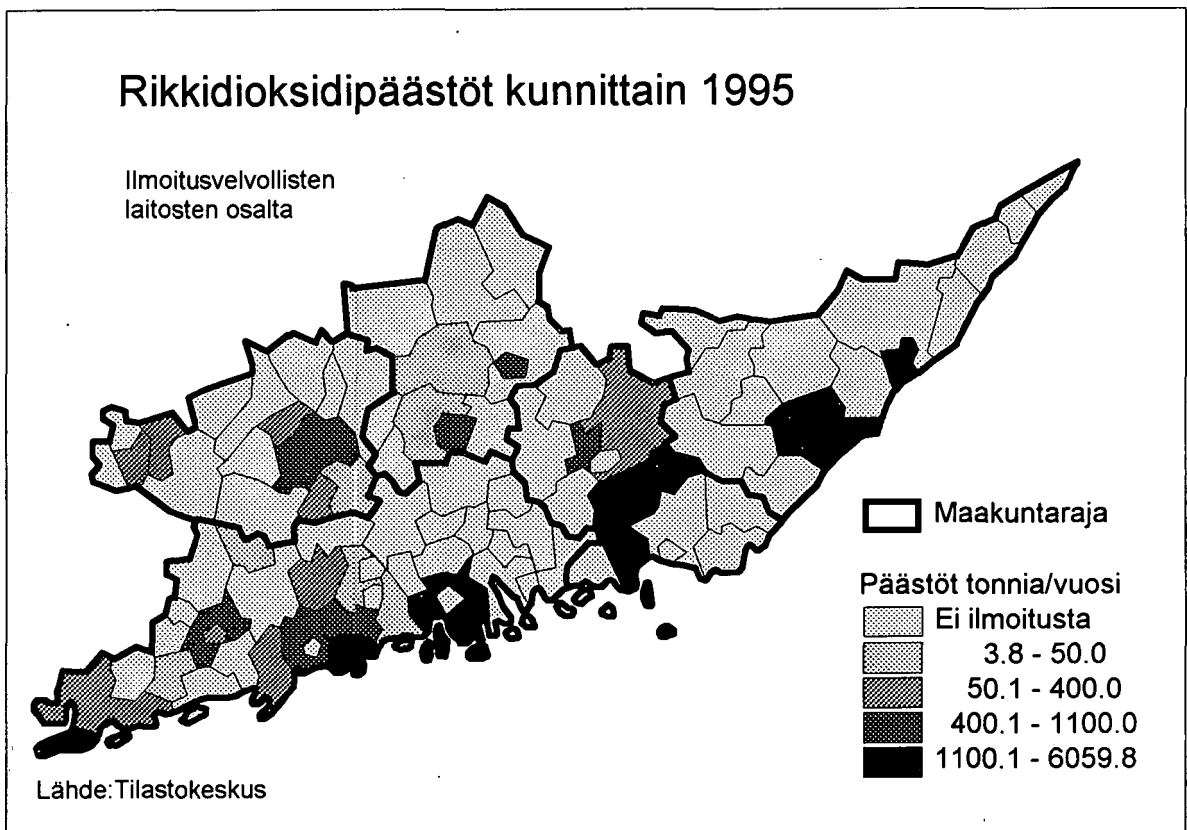
Kuva 127. Rikkidioksidipäästöt ( \text{SO}_2 ) kunnittain 1995.
