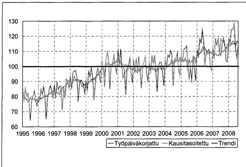
Kuvio 8. Kemianteollisuus TOL 23-25, teollisuustuotannon volyyymi-indeksi 1995 – 2008 elokuu, 2000=100
