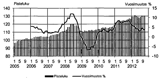
Maarakennusalan konekustannusindeksi 2005=100
