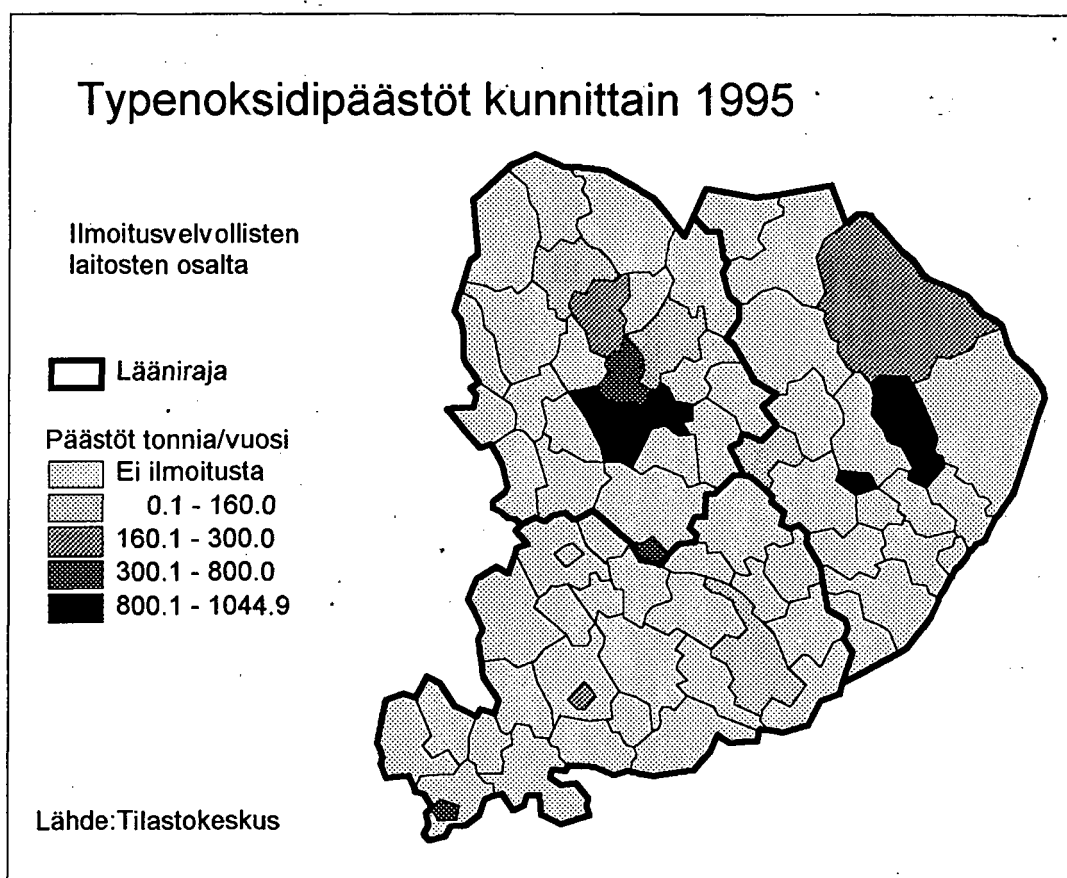
Kuva 128. Typen oksidipäästöt ( \text{NO}_x ) kunnittain 1995.
