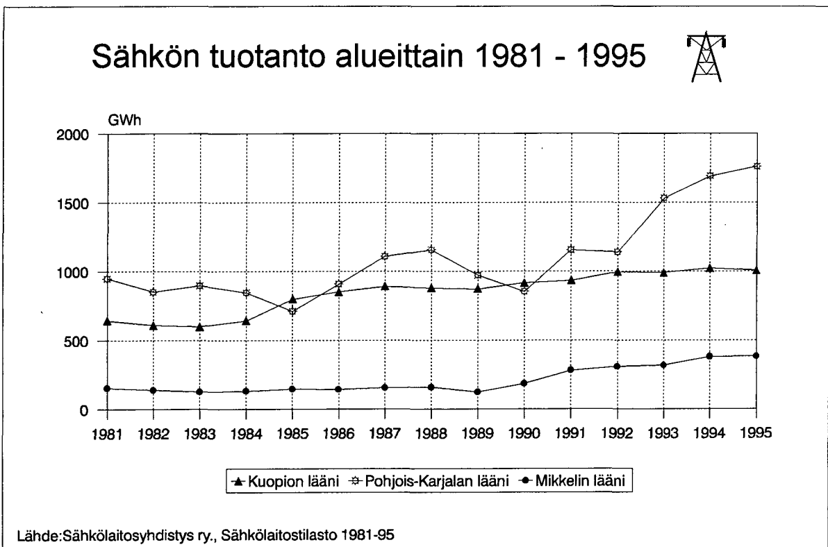
Kuva 118. Sähkön tuotanto alueittain 1981 - 1995.
