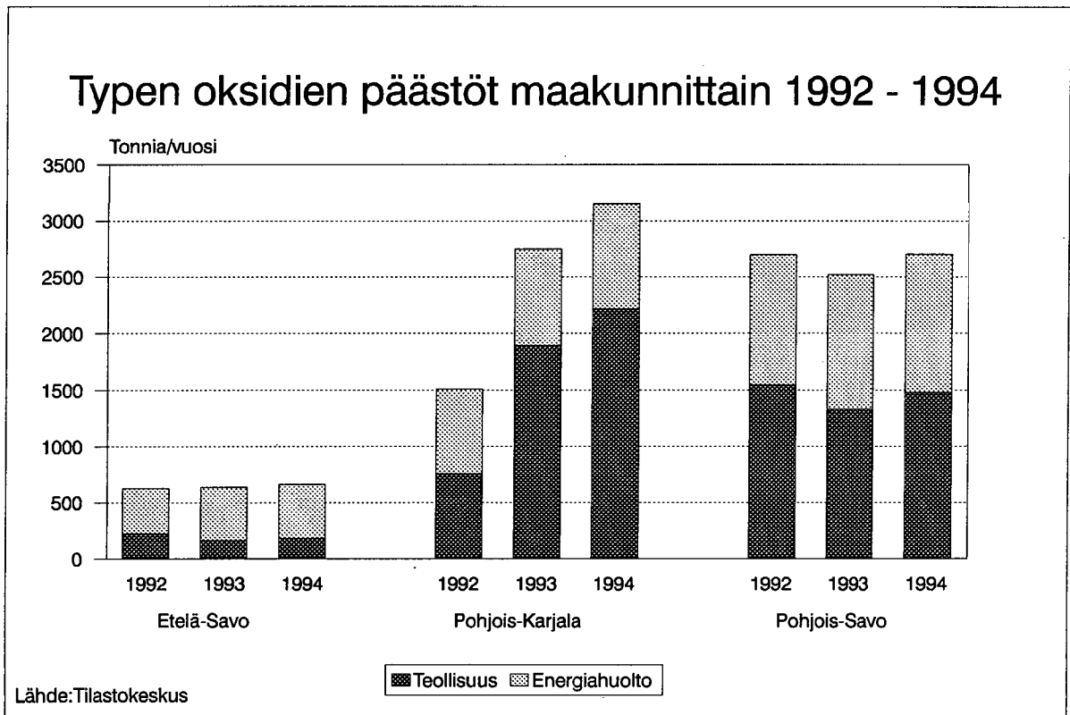
Kuva 125. Typen oksidien päästöt maakunnittain 1992 - 1994.
