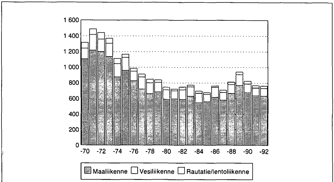
Kuvio 7 Liikenteessä kuolleet kuolemansyytilaston mukaan 1970 – 1992
