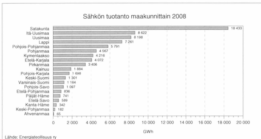
Kuva 4.3. Sähkön tuotanto maakunnittain 2008.
