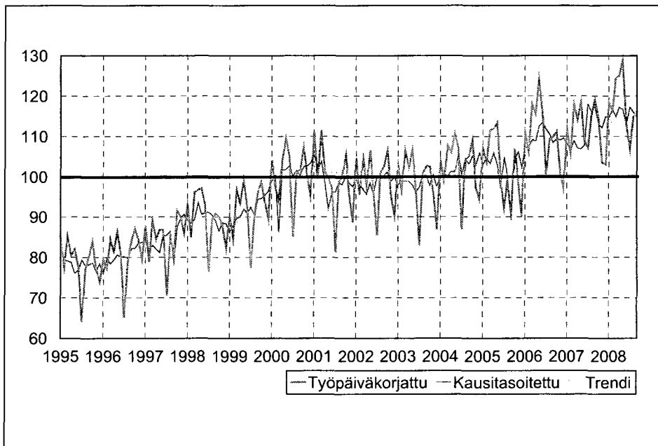
Kuvio 8. Kemianteollisuus TOL 23-25, teollisuustuotannon volyyymi-indeksi 1995 – 2008 syyskuu, 2000=100
