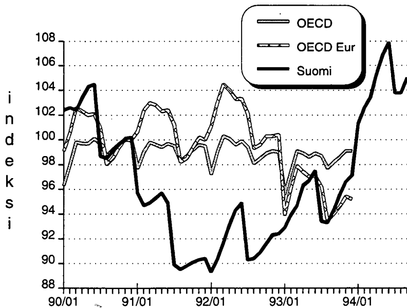
Kuvio 4. Teollisuuden volyymin muutos (C, D, E) Suomi, OECD ja OECD Eurooppa (1990=100, kumulatiivinen työpäiväkorjattu tammi-syyskuu)
