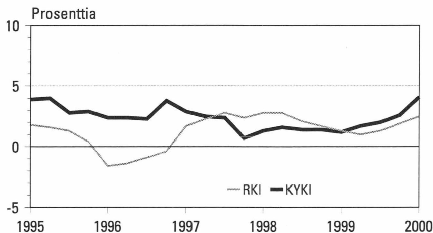
Kiinteistön ylläpidon kustannusindeksin 1995=100 ja rakennuskustannusindeksin 1995=100 vuosimuutokset
