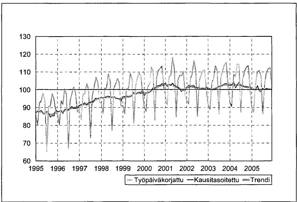
Kuvio 6. Muu tehdasteollisuus TOL 15, 17, 18, 19, 22, 26, 36, 37 teollisuustuotannon volyyymi-indeksi 1995 – 2005, 2000=100
