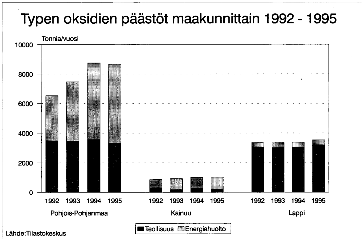
Kuva 117. Typen oksidien päästöt maakunnittain 1992 - 1995.
