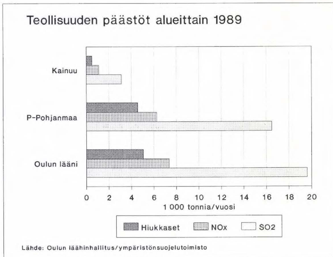
Kuva 91. Teollisuuden päästöt alueittain 1989.
