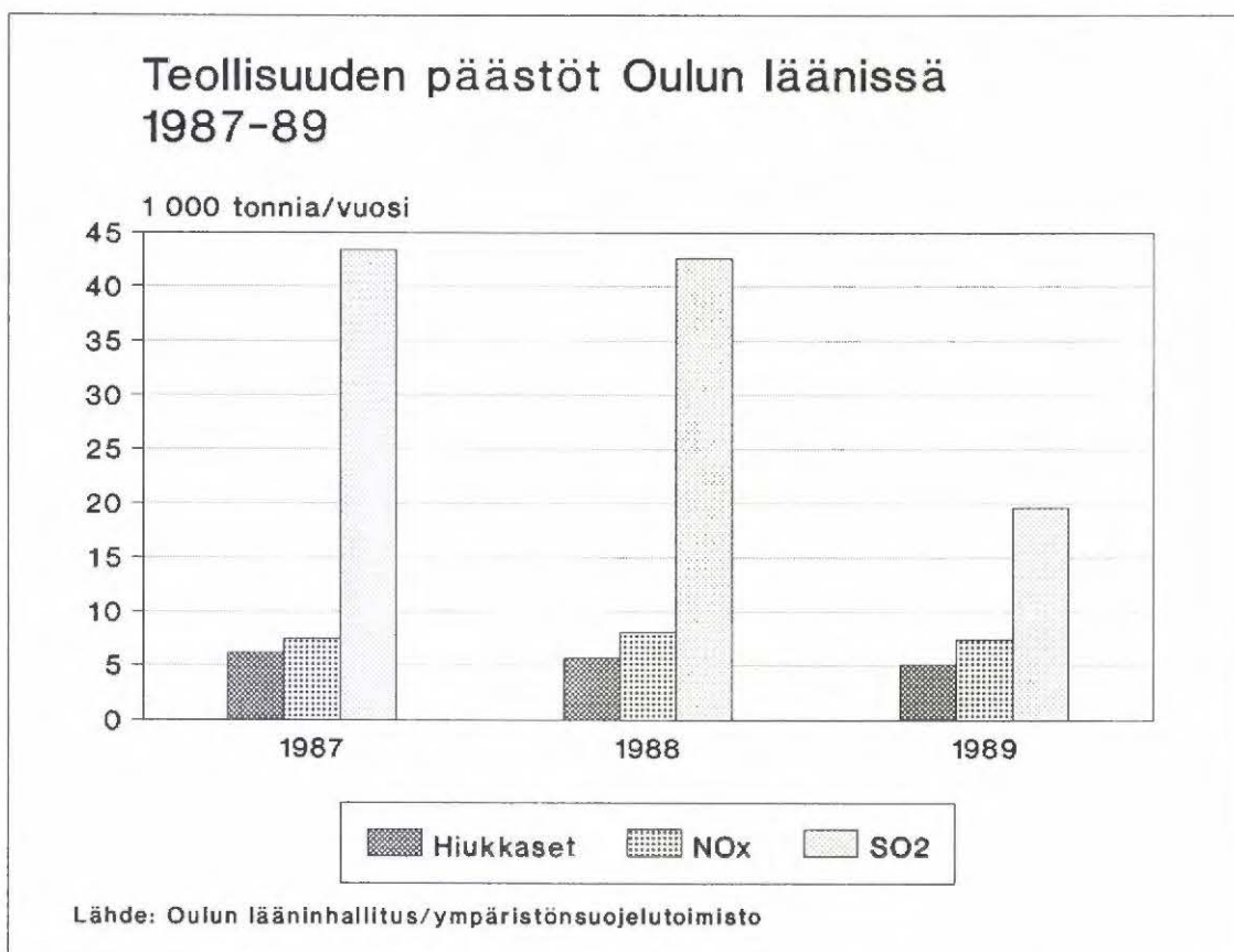
Kuva 94. Teollisuuden päästöt Oulun läänissä 1987-89.
