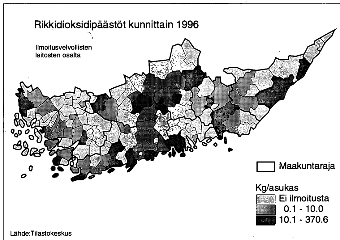
Kuva 120. Rikkidioksidipäästöt ( \text{SO}_2 ) kunnittain 1996.
