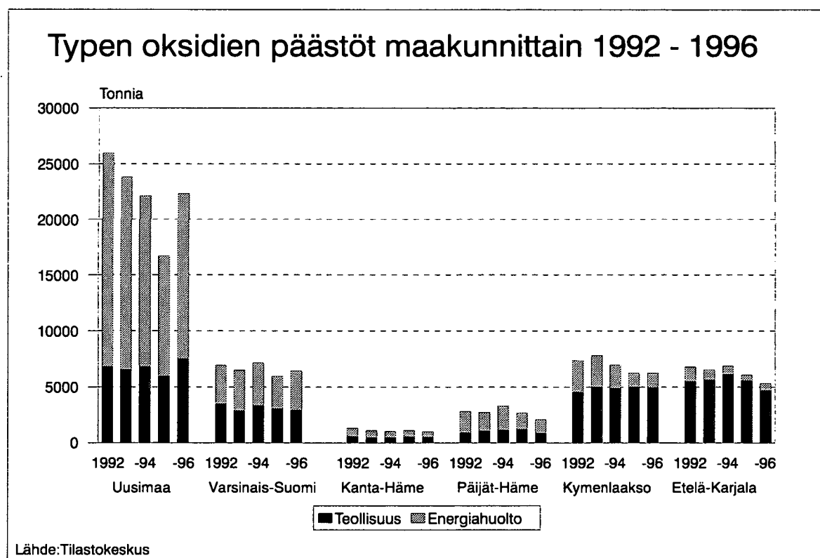
Kuva 116. Typen oksidien päästöt maakunnittain 1992 - 1996.
