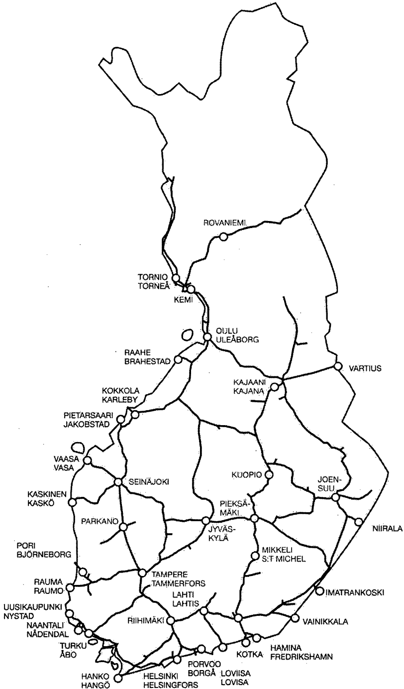
Kuvio 6 – Figure 6 Suomen rataverkko, 2000 Railway network, 2000
