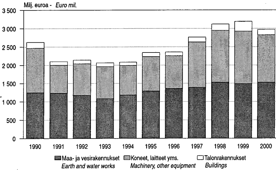
Kuvio 2 - Figure 2 Liikenteen ja viestinnän investoinnit, 1990 - 2000 Transport and communication investments, 1990 - 2000
