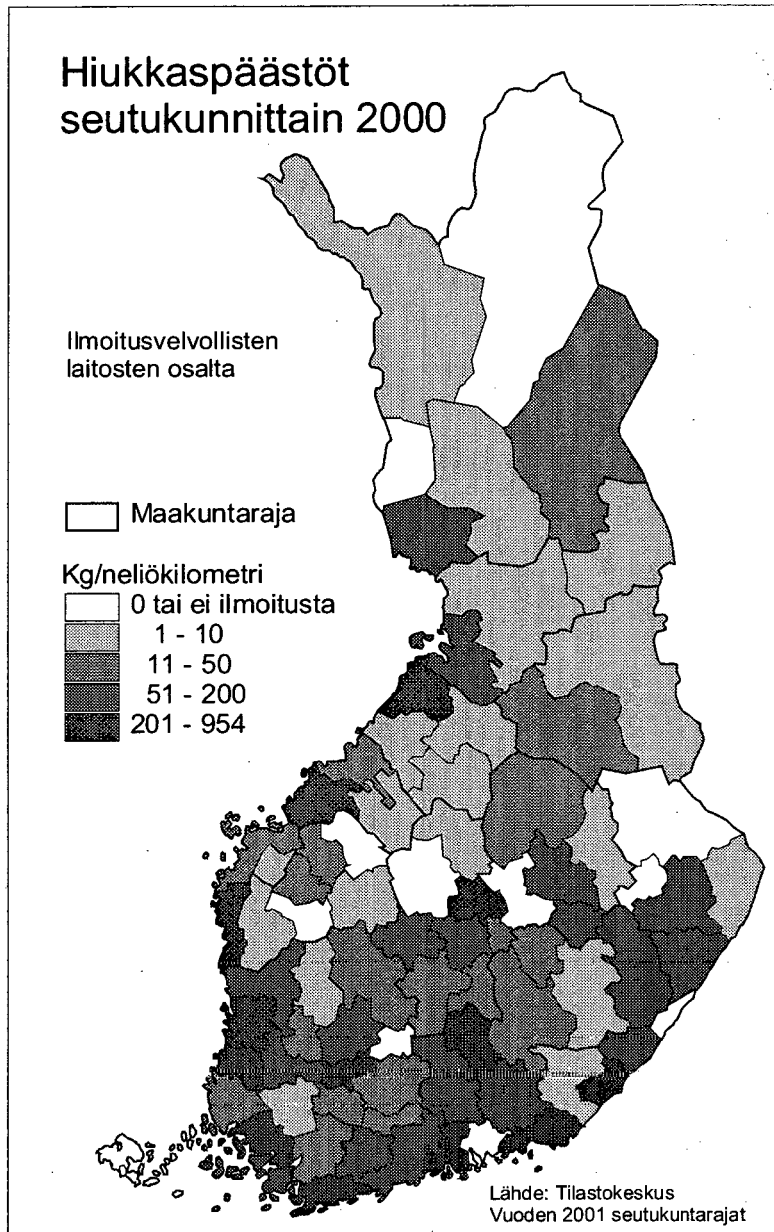
Kuva 194. Hiukkaspäästöt seutukunnittain 2000.
