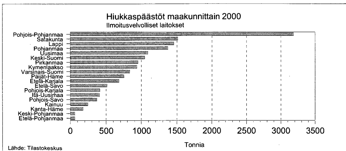
Kuva 195. Hiukkaspäästöt maakunnittain 2000.
