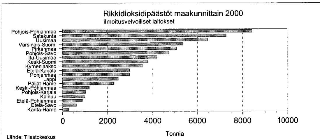
Kuva 197. Rikkidioksidipäästöt maakunnittain 2000.
