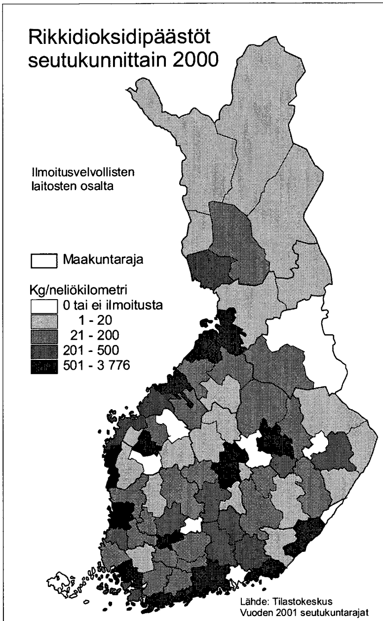
Kuva 196. Rikkidioksidipäästöt seutukunnittain 2000.
