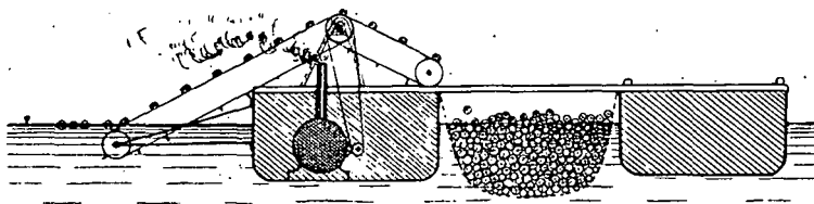
Ångknipningsverk invid Haapakoski.
