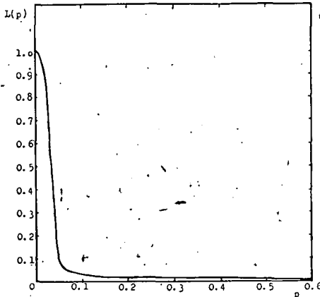
Kuvio 1. OC-käyrä — Figur 1. OC-kurva Figure 1. OC Curve
