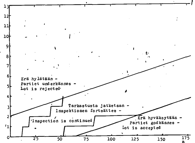
Kuvio 2. Päätösalueet — Figur 2. Beslutsområden Figure 2. Decision areas
