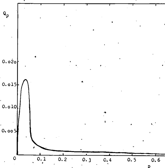
Kuvio 4. AOQ-käyrä — Figur 4. AOQ-kurva Figure 4. AOQ Curve
