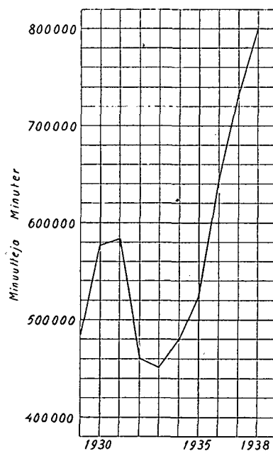
Diagr. XII. Suomen Ruotsin puhelinkaapelin kuormitus vuosina 1929—1938. Belastningen å telefonkabeln Finland Sverige åren 1929—1938.
