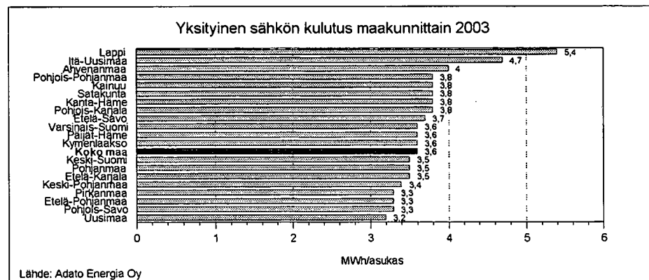
Kuva 4.10. Yksityinen sähkön kulutus maakunnittain 2003.
