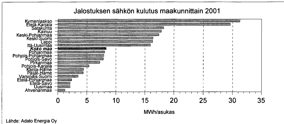
Kuva 184. Jalostuksen sähkön kulutus maakunnittain 2001.
