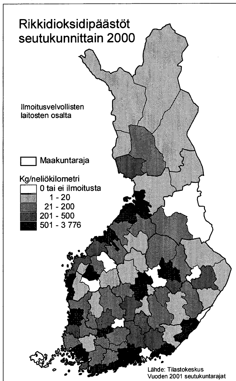
Kuva 194. Rikkidioksidipäästöt seutukunnittain 2000.
