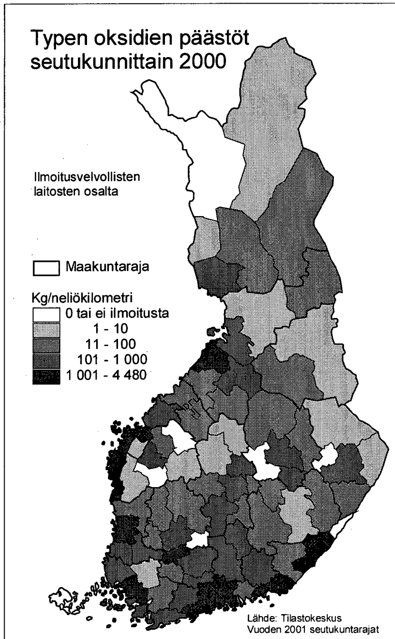
Kuva 190. Typen oksidien päästöt seutukunnittain 2000.
