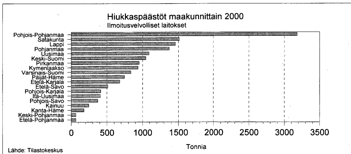
Kuva 193. Hiukkaspäästöt maakunnittain 2000.
