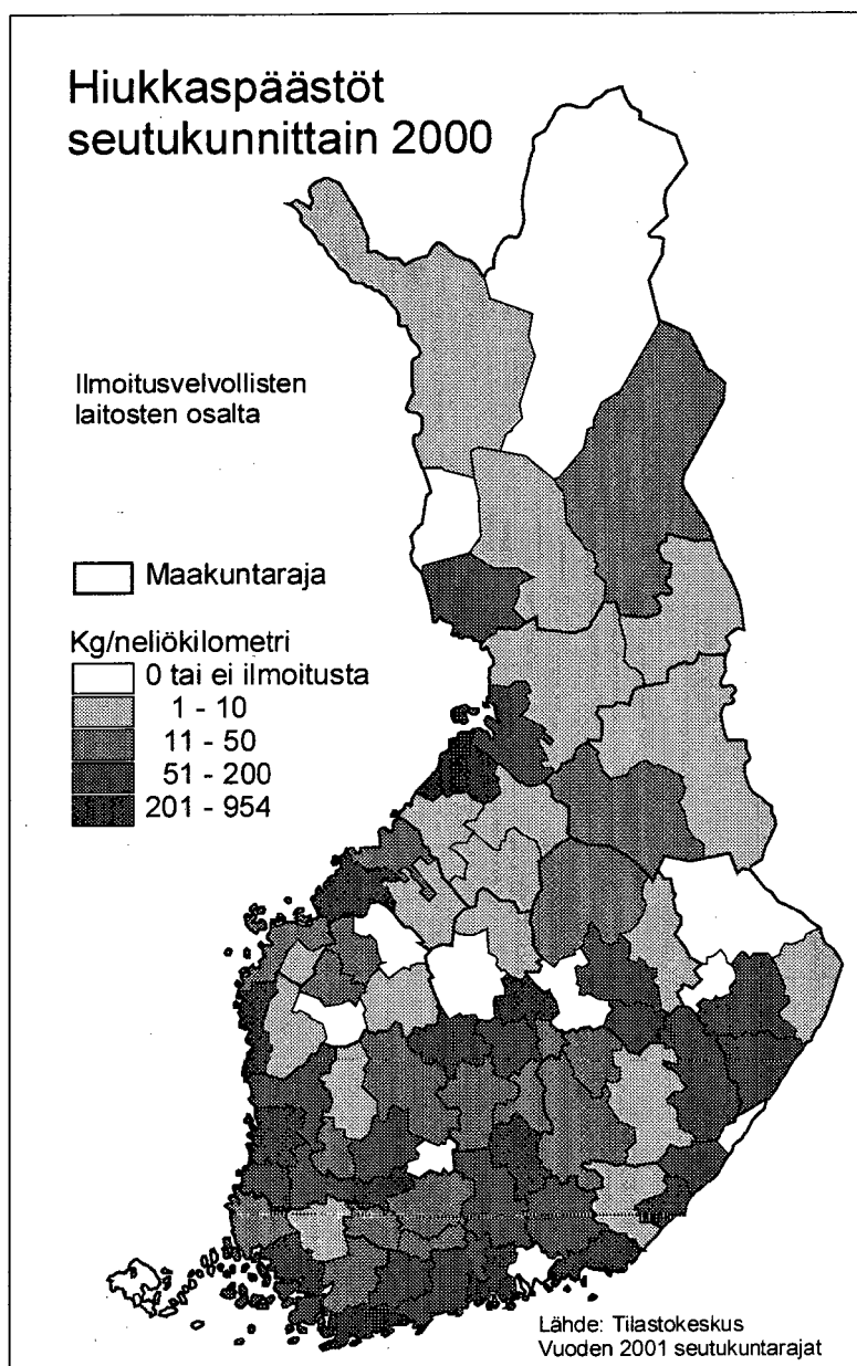
Kuva 192. Hiukkaspäästöt seutukunnittain 2000.
