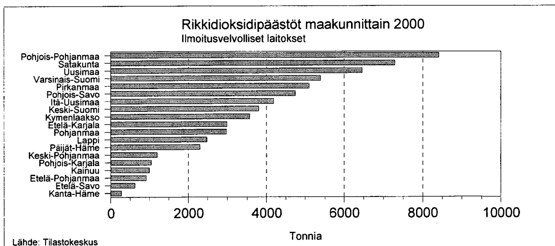
Kuva 195. Rikkidioksidipäästöt maakunnittain 2000.
