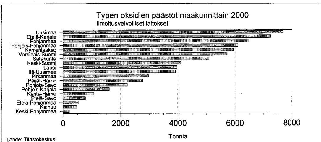
Kuva 191. Typen oksidien päästöt maakunnittain 2000.
