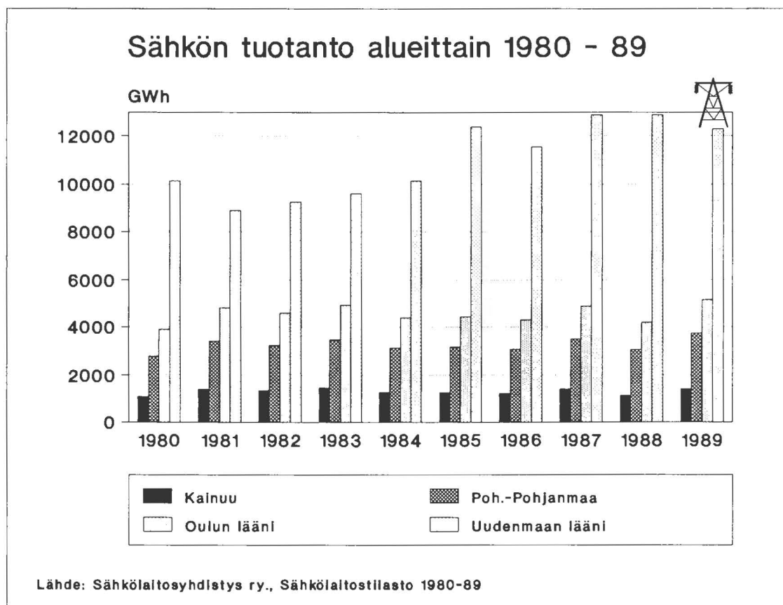
Kuva 93. Sähkön tuotanto alueittain 1980-89.
