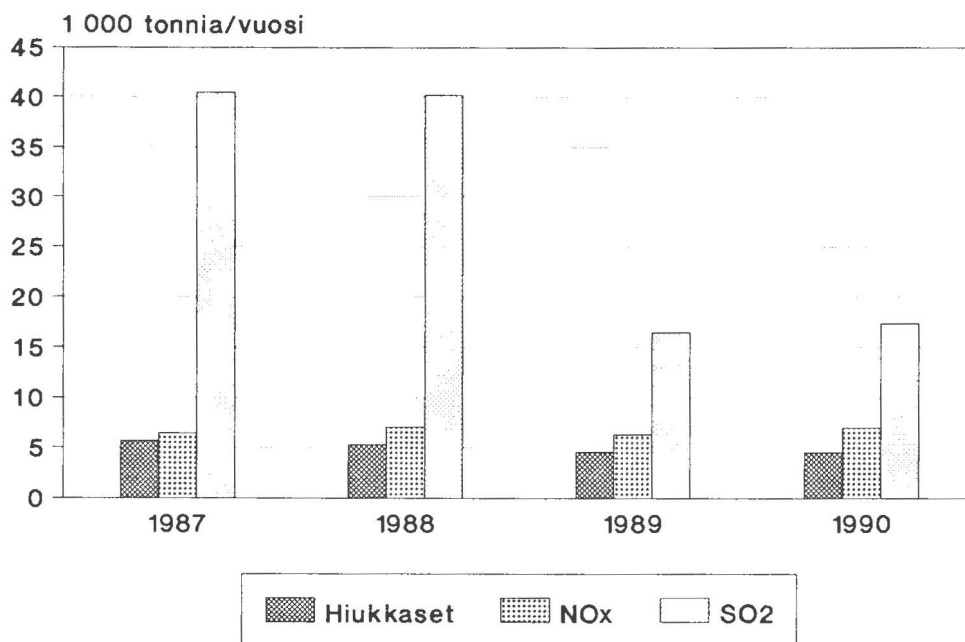
Kuva 102. Teollisuuden päästöt Pohjois-Pohjanmaalla 1987-1990.
