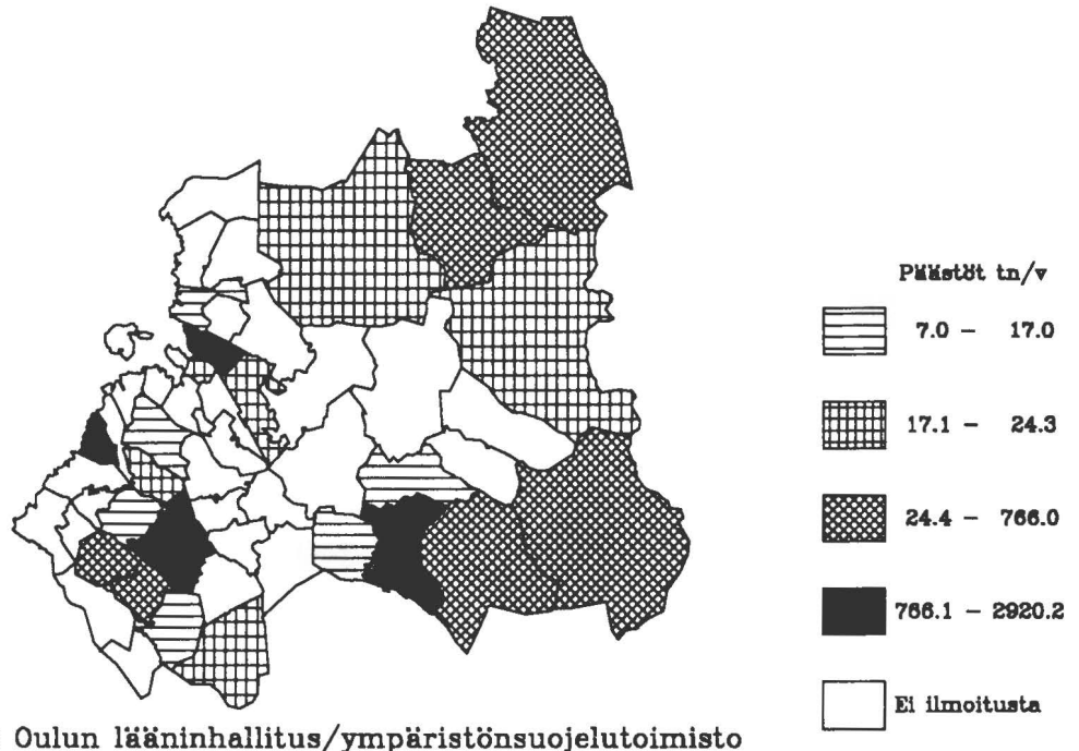
Kuva 107. Typpidioksidipäästöt kunnittain ilmoitusvelvollisten osalta 1990 (tonnia/vuosi).
