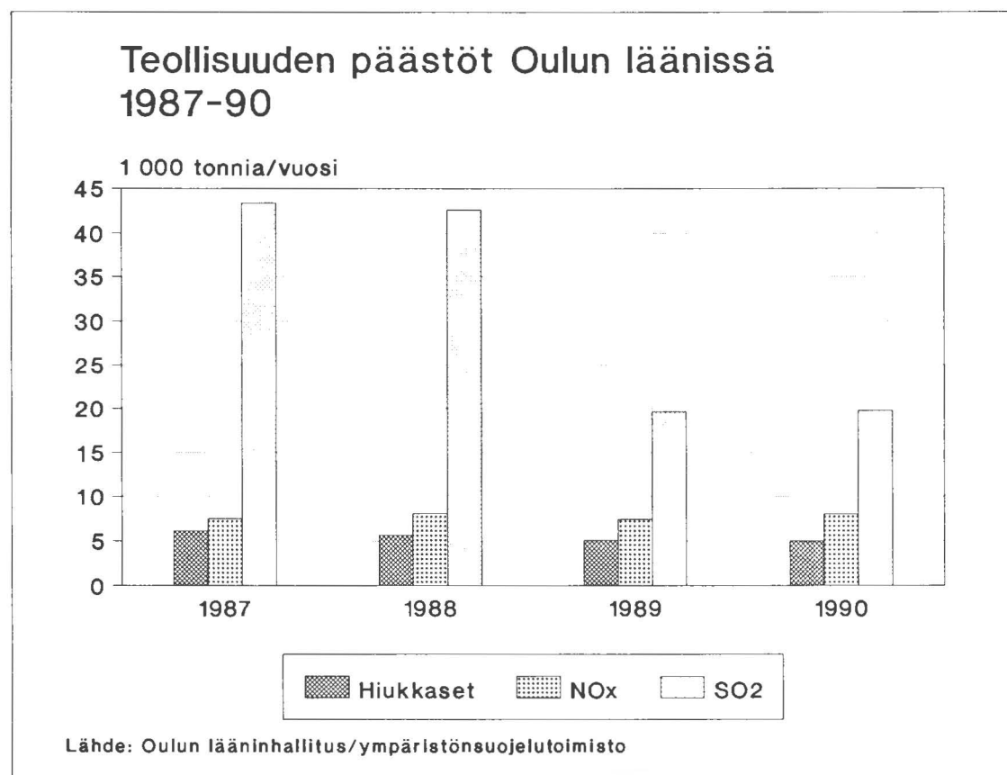
Kuva 104. Teollisuuden päästöt Oulun läänissä 1987-90.
