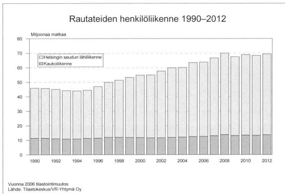
Kuva 7.5. Rautateiden henkilöliikenne 1990–2012.
