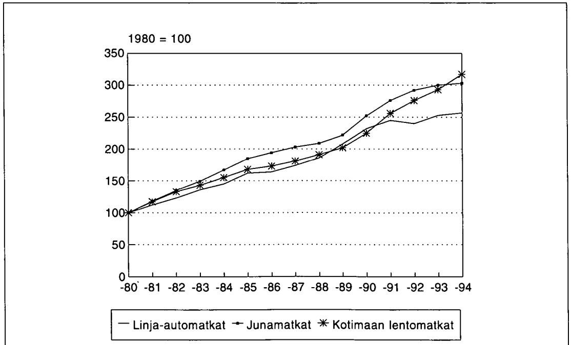
Kuvio 6 Pitkien linja-automatkojen, junamatkojen ja kotimaan lentomatkojen hintakehitys 1980 – 1994 (1980=100)
