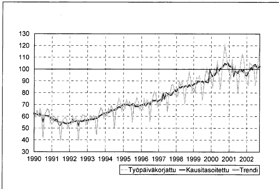
Kuvio 5. Koko teollisuus TOL C,D,E, teollisuustuotannon volyymi-indeksi 1990 – 2002 lokakuu, 2000=100
