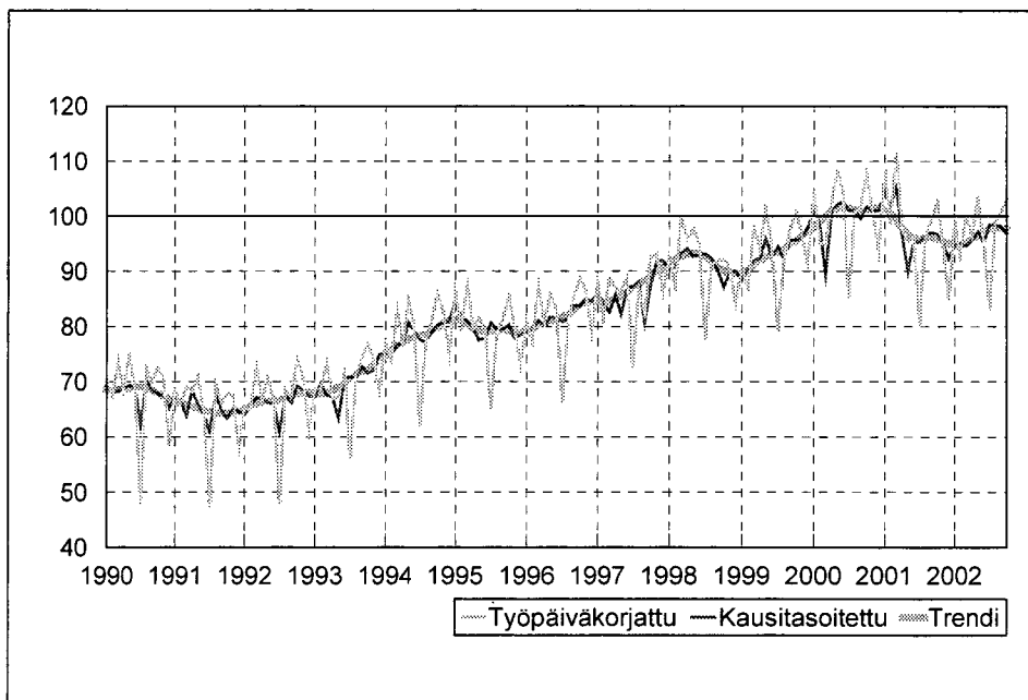
Kuvio 8. Kemian teollisuus TOL 23-25, teollisuustuotannon volyyymi-indeksi 1990 – 2002 lokakuu, 2000=100
